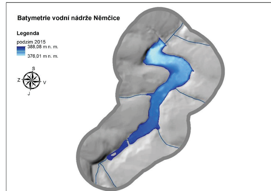
Obr. 2: DMR VN Némčice (2015) zdroj dat River Surveyor M9
