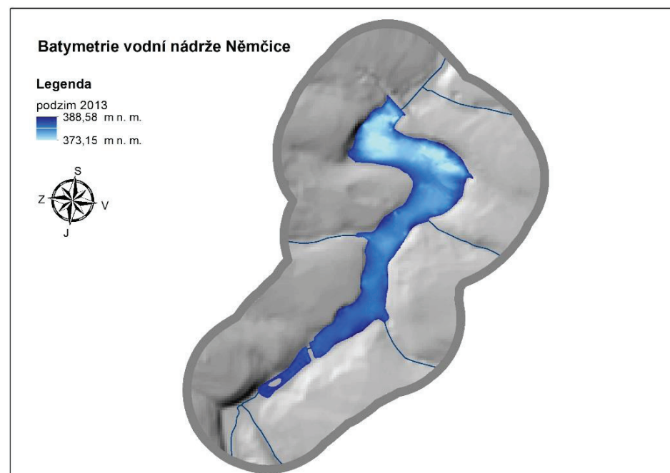
Obr. 1: DMR VN Némčice (2013) zdroj dat JOSKA (PVL)
