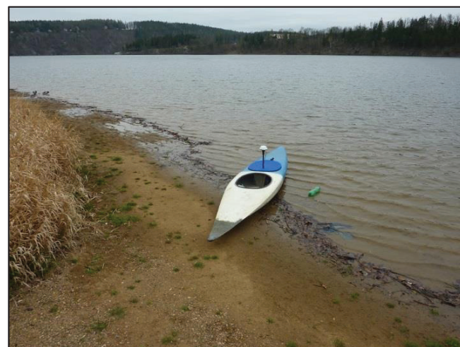
Foto č. 1: River Surveyor M9 osazený na kayak
